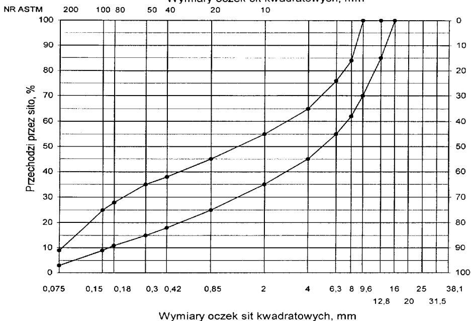
Rys. 10. Krzywe graniczne uziarnienia mieszanki mineralnej BA od 0 do 12.8mm do warstwy wiążącej, wyrównawczej i wzmacniającej nawierzchni drogi o obciążeniu
