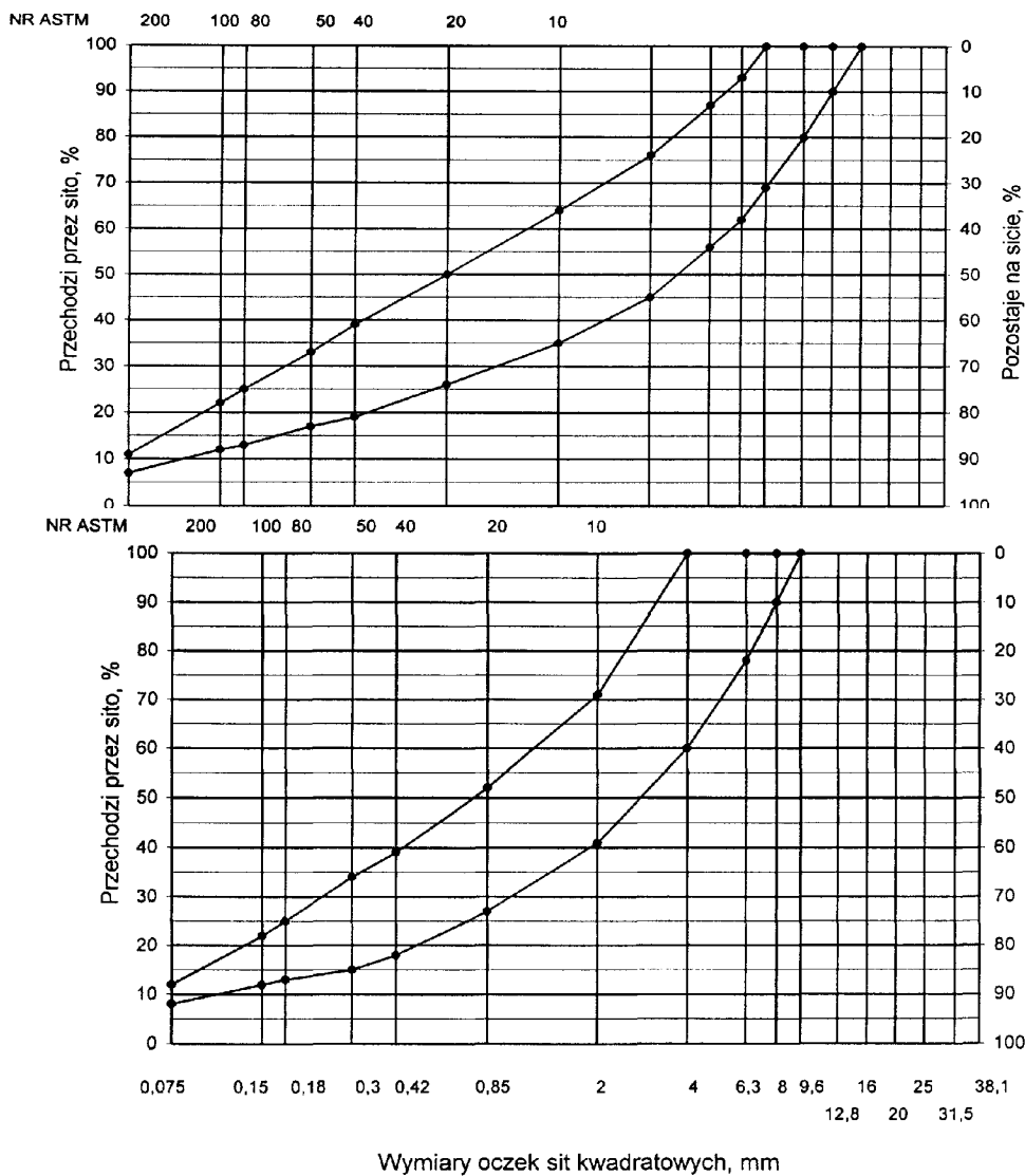
Rys. 2. Krzywe graniczne uziarnienia mieszanki mineralnej BA od 0 do 16mm, od 0 do 12.8mm do warstwy ścieralnej nawierzchni drogi o obciążeniu ruchem KR1 lub KR2
